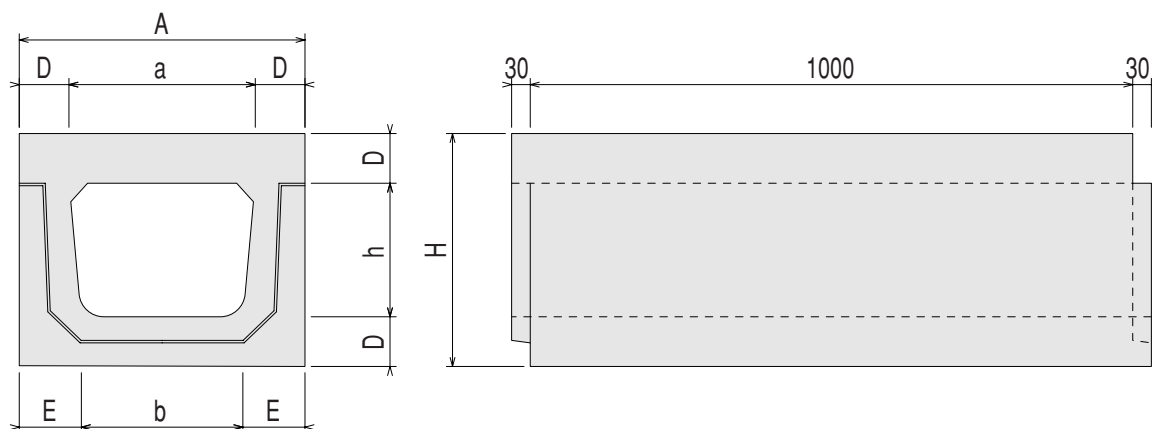
形状寸法図
